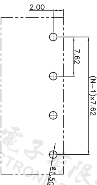
P.C.B. LAYOUT
