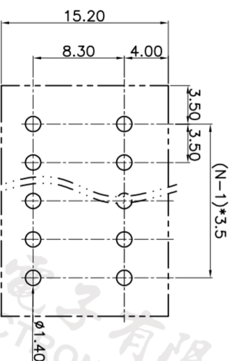
P.C.B. LAYOUT
