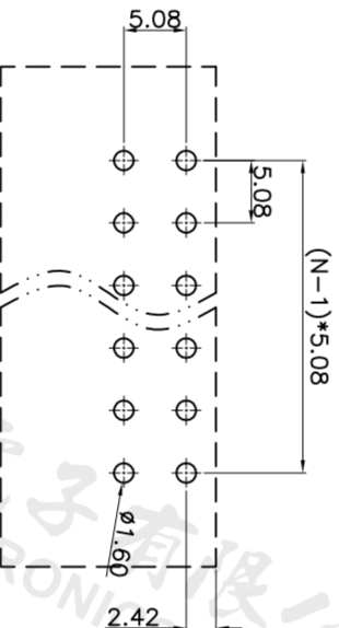
P.C.B. LAYOUT
